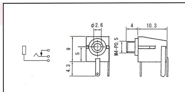
◆φ2.5 モノラルジャック パネル
